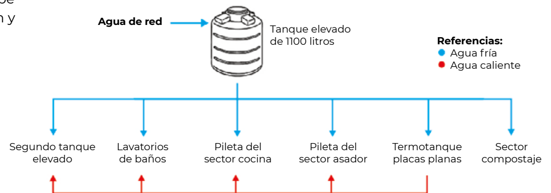
Esquema de abastecimiento de agua de red fría y caliente del SUME.
