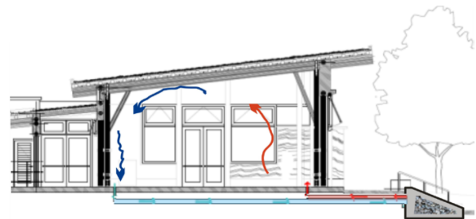
Corte de esquema de funcionamiento de los lechos de piedras.
