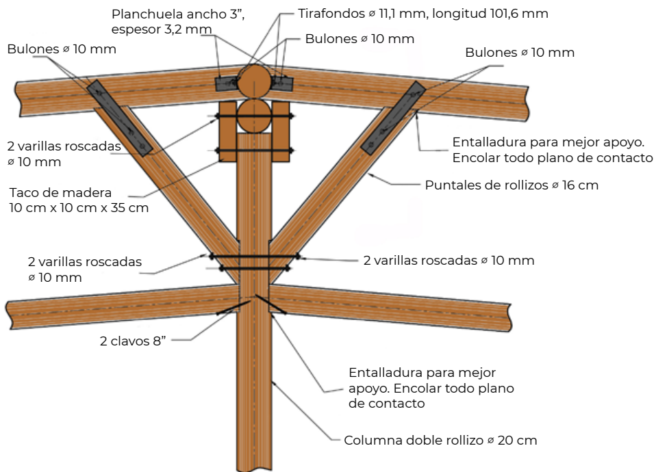
Unión de pórtico longitudinal con sus medios de unión reforzados con la utilización de cola adhesiva en los planos de contacto.
