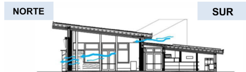
Corte del salón principal con esquema de ventilación cruzada.
