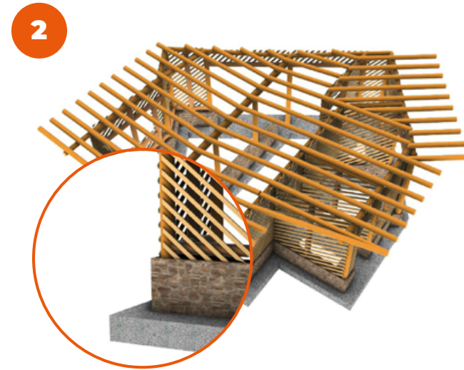
Entramado de madera en muros y estructura de cubierta.
