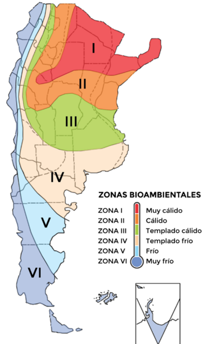
Zonas bioambientales de la República Argentina. Basado en norma IRAM 11603.
