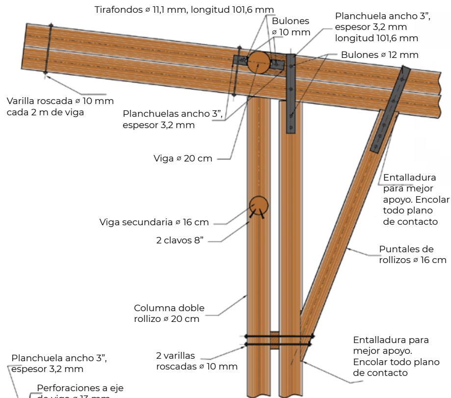
Unión de vigas dobles y columnas dobles con puntales de los pórticos transversales. Se utilizan planchuelas, bulones, varillas roscadas y clavos espiralados.
