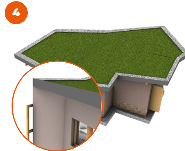
Revestimiento de tierra y techo vivo.
