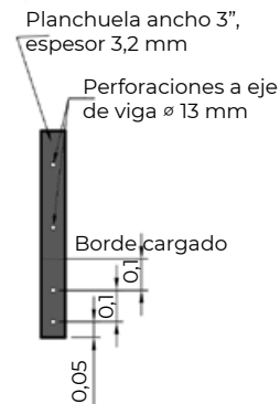
Unión de vigas y columnas dobles. Se utilizan bulones y planchuelas metálicas para garantizar la transferencia de esfuerzos.
