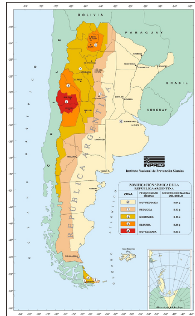
Mapa de zonificación sísmica de Argentina. Fuente: Instituto Nacional de Prevención Sísmica.
